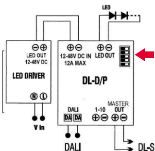
Schema di collegamento DALI Wiring diagram DALI
